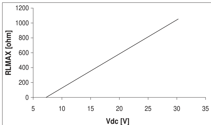
Fig. 3 Resistenza di carico in funzione della tensione di alimentazione.
